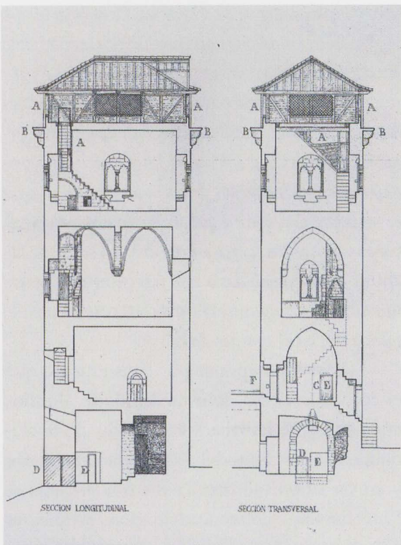
Torre de Hércules (sección). (Ministerio de Obras Públicas y Urbanismo, 1981)
