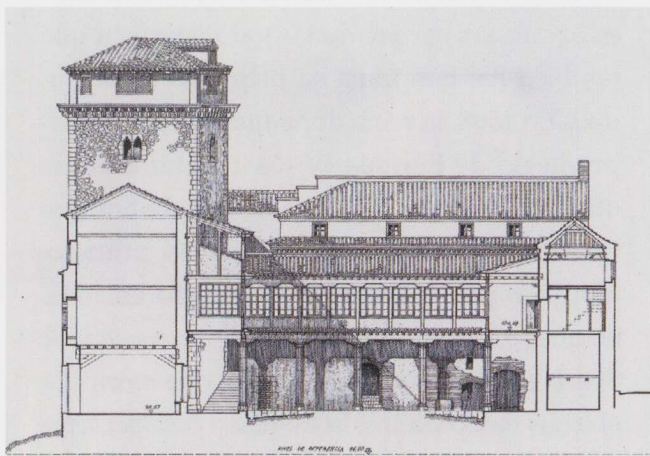
Sección del convento de Santo Domingo. (Ministerio de Obras Públicas y Urbanismo, 1981)
